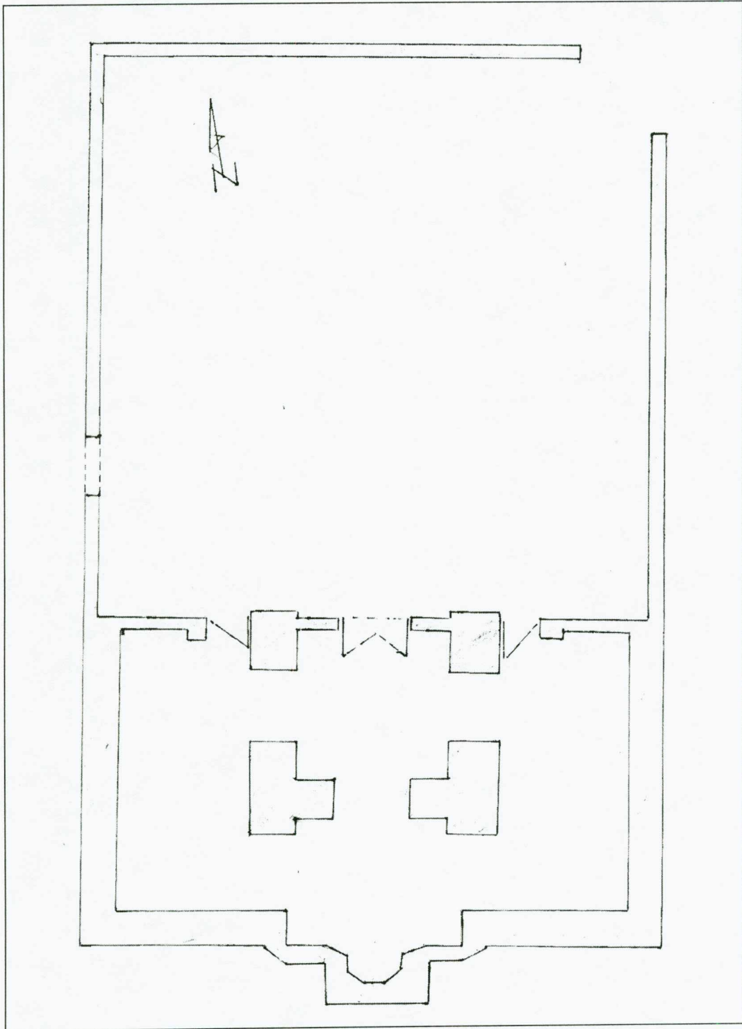
پلان مسجد جامع چنار، مقیاس ۱/۱۰۰
